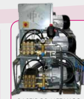
BASTIDOR METALICO BOMBAS
